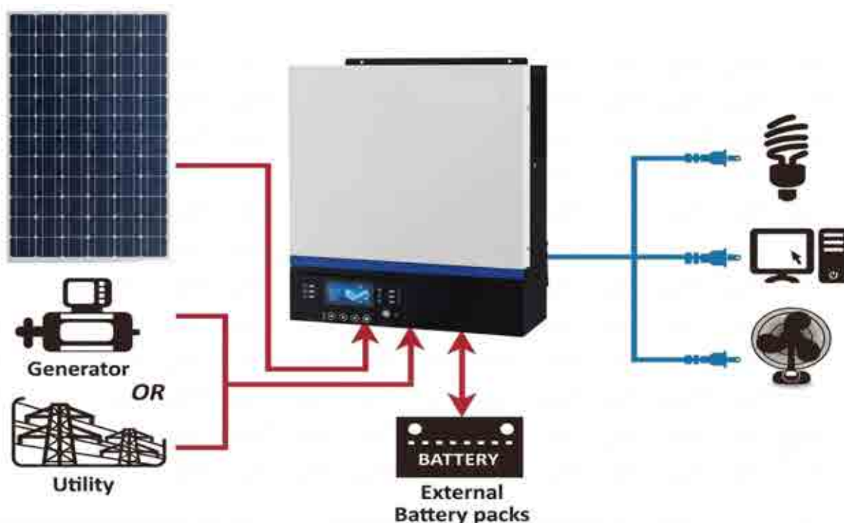
Figura 1. Funcionamiento del sistema fotovoltaico
