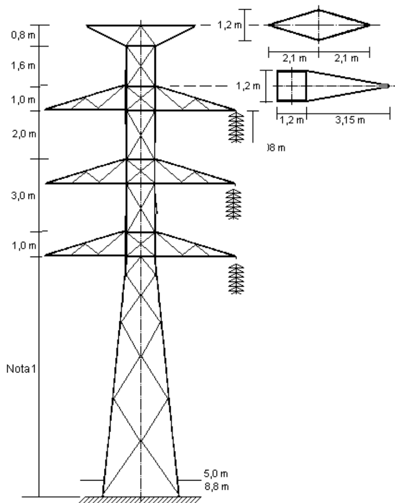
Figura 1. Torres modeladas a 115, 230 y 400 kV.
